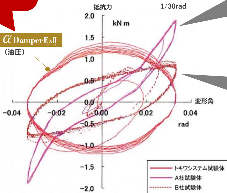
基本性能曲線（リサーチ曲線）
